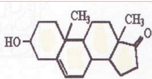
DHEA MOLECULE
